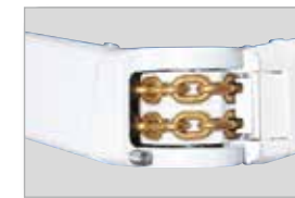
La double chaîne à maillons en acier rond est logée dans les bras articulés et est ainsi protégée contre la corrosion.
