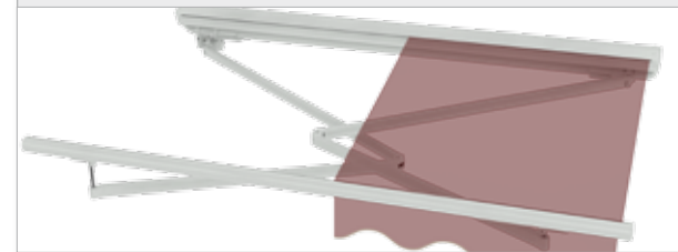
Bras croisés lors de la phase d'extension.
