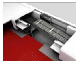
Vue de coupe - rail de guidage avec système zip et profilé en plastique à l'intérieur et courroie en tissu élastique.
