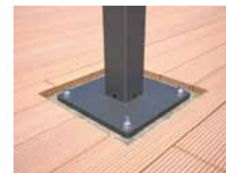
Markisenständer mit Fußplatte zum Aufschrauben auf ein Betonfundament.
